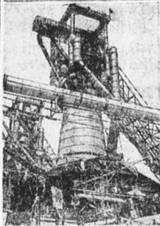
Домна № 1 Керченского металлургического завода 20 апреля с. г. выпустила первую партию чугуна.
